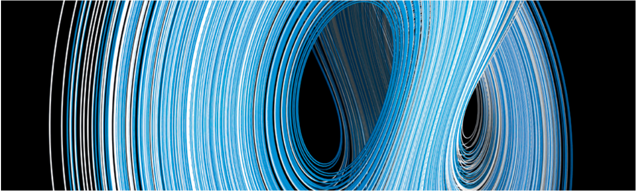
Bild: Lorenz-Attraktor von Jos Leys
